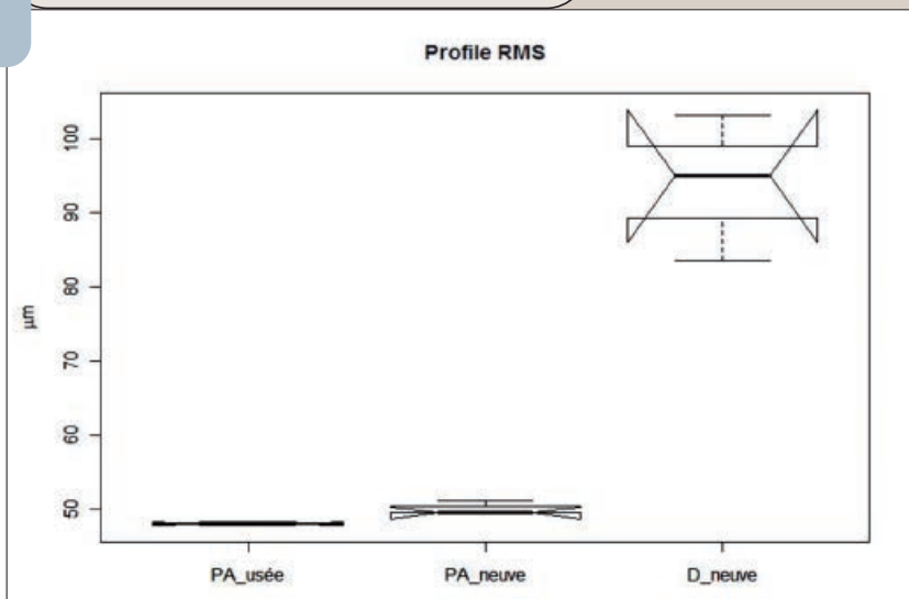
Figure 4. Valeurs moyennes des écarts-types des profils longitudinaux mesurés sur du pin d'Alep usiné avec un outil à arête émoussée (PA usée), du pin d'Alep avec un outil à arête neuve (PA neuve) et du pin Douglas avec un outil neuf (D neuve).
