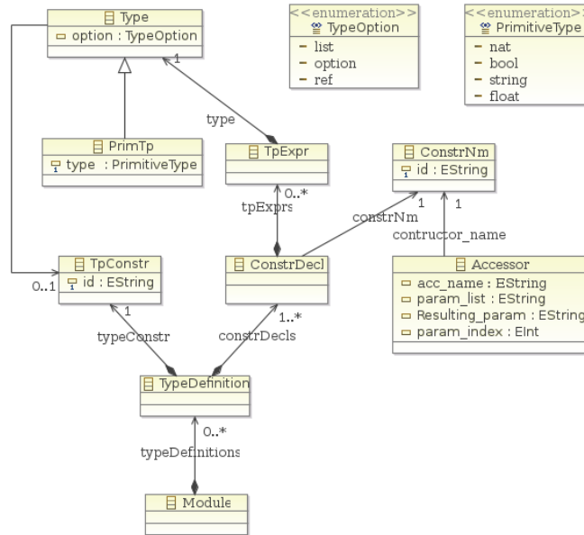
Fig. 3. Datatype Meta-model
