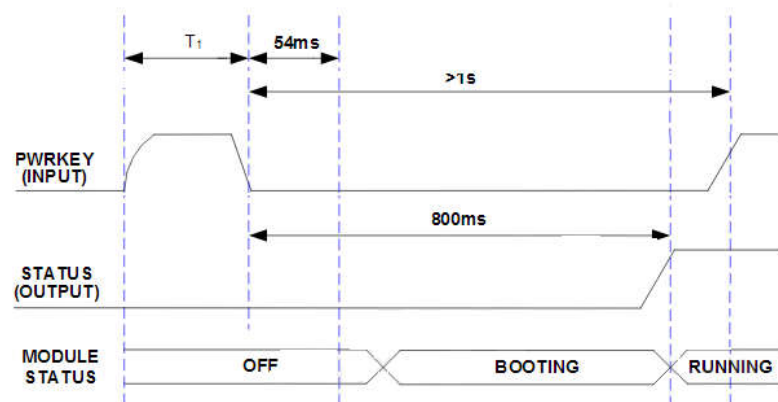
Figure IV.6: Cycle de démarrage de Module GPRS [31]
